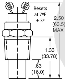
BULBO FAN CLUTCH 180 NO
