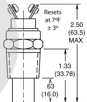
BULBO FAN CLUTCH 185 NO
