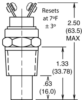
BULBO FAN CLUTCH 200 NC
