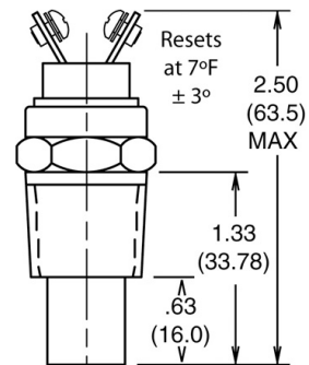
BULBO FAN CLUTCH 205 NC
