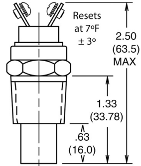
BULBO FAN CLUTCH 195 NC
