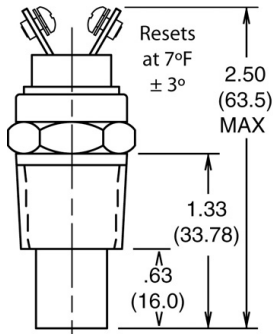
BULBO FAN CLUTCH 190 NC
