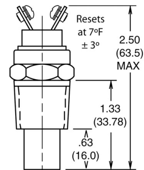
BULBO FAN CLUTCH 185 NC
